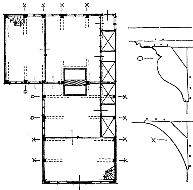
Reconstructie van het huis Westzijde 185 te Zaandam.
