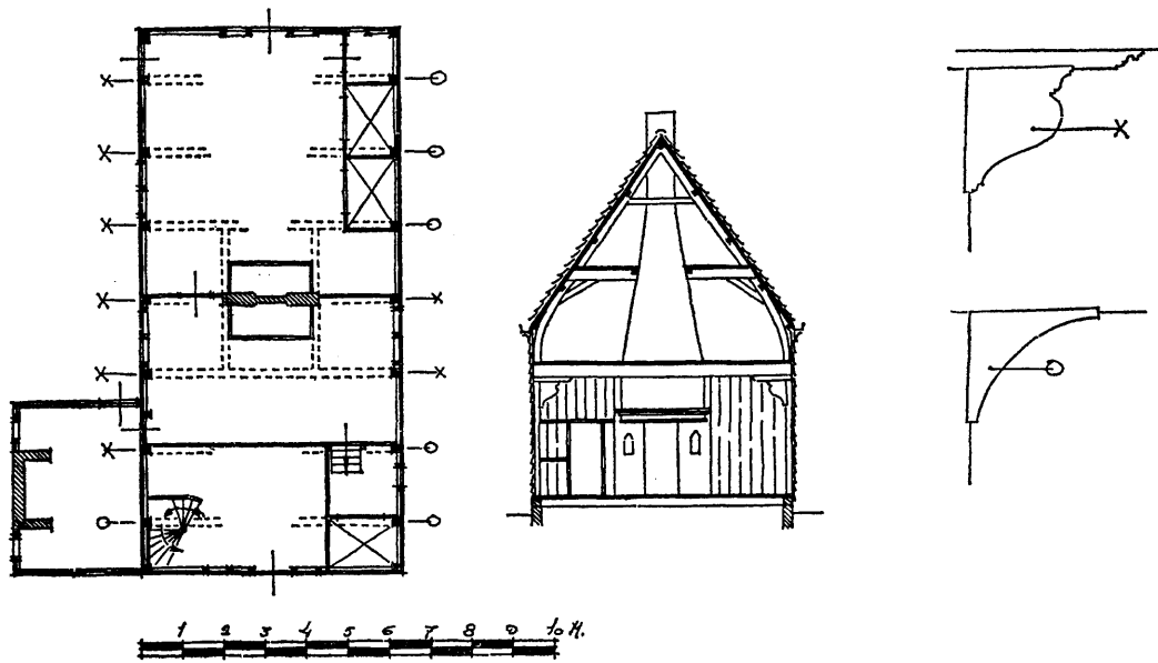
Reconstructie van het huis Jagerspad 1 te Zaandam.
