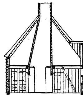
DOORSNEDEN B-B
