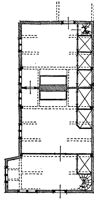
Reconstructie van het huis Hogendijk 62 te Zaandam (Tekening H. J. Zantkuyl)
