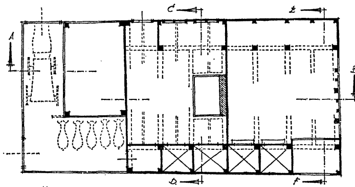
PLATTEGROND.
