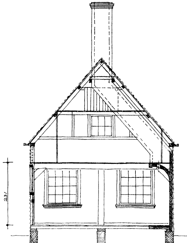
doorsnede CD.
